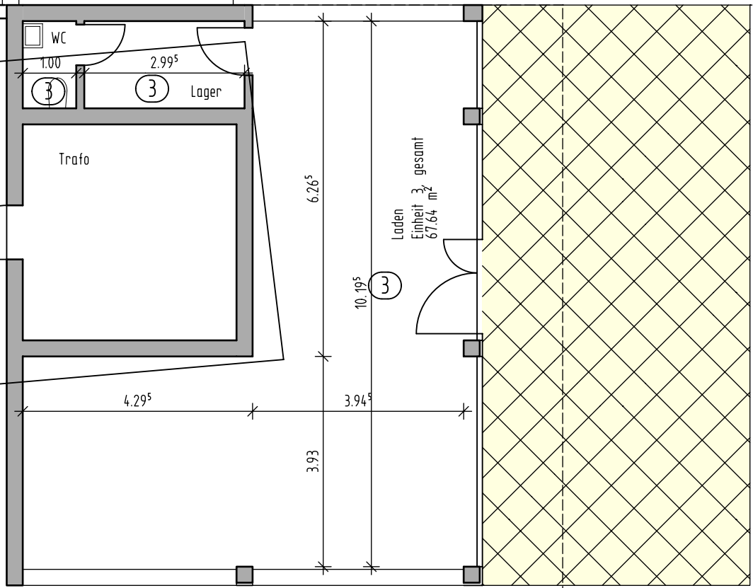
Schnitt Nebengebäude
